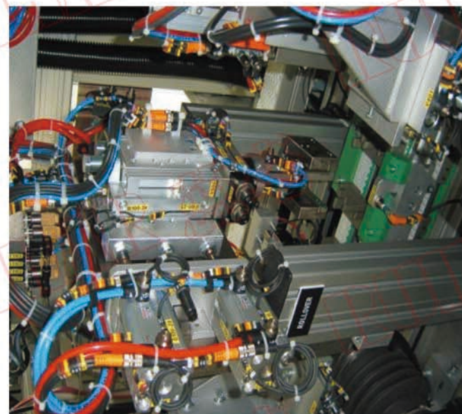
配件自动组装机
