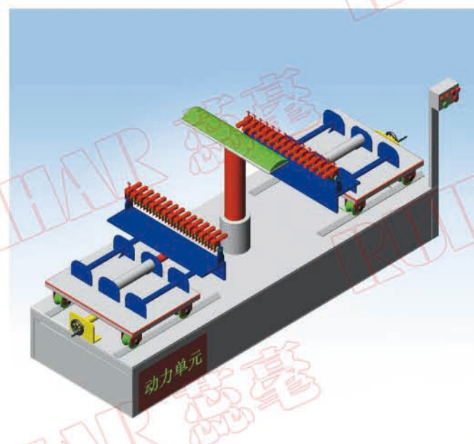
钢板弯曲成型夹具系统
