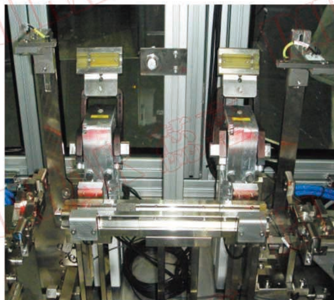
自动压装工作台
